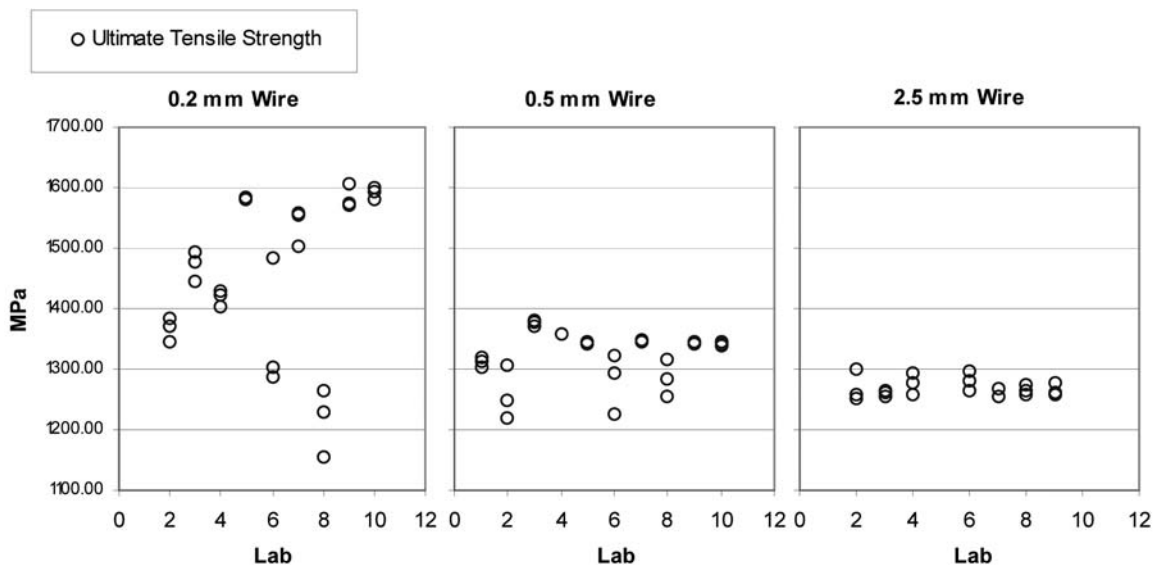
FIG. X2.4 Ultimate Tensile Strength
